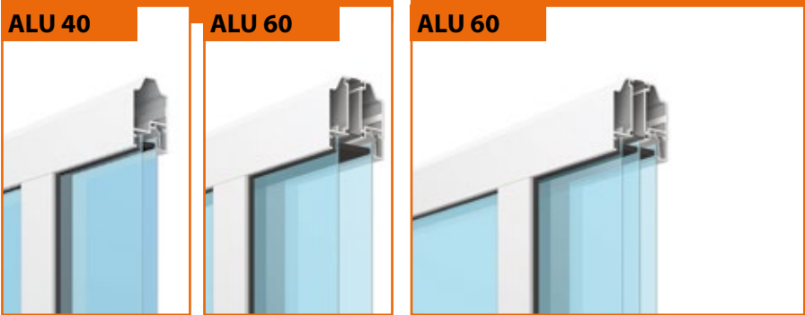
Doppelwandig transparente Füllung (20 mm) in: Acrylglas, Polycarbonat, Plexiglas (100 % Lichtdurchlässigkeit) (40 mm) in: Acrylglas, Polycarbonat, Plexiglas (100 % Lichtdurchlässigkeit)
