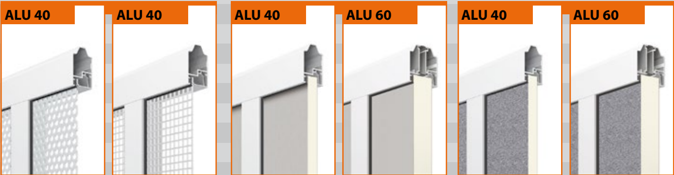
Einwandig, perforiertes Aluminiumblech (2 mm) rund perforiert (40 % Luftdurchlässigkeit) (2 mm) quadratisch perforiert (70 % Luftdurchlässigkeit)
